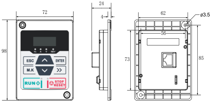
(c) A90-4T060KEY2 外引键盘外形
