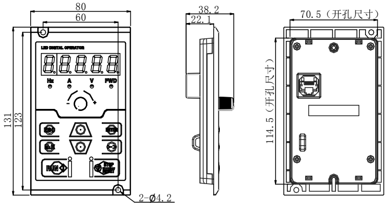
(d) A90-4T060KEY3 外引键盘外形
