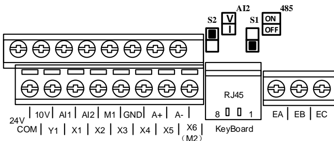
图 3-5 控制回路端子排列
