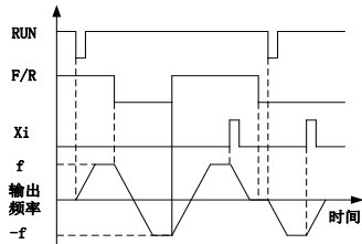
(c) F00.03=3 三线控制接线示意图 (d) F04.19=0, F00.03=3 正/反转运行逻辑图 图 5-3 三线控制
