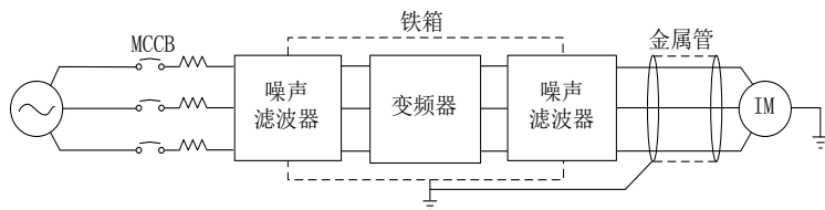
图 3-4 减少对外干扰的对策
