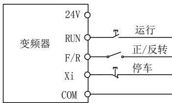
(c) F00.03=3 三线控制接线示意图 (d) F04.19=0, F00.03=3 正/反转运行逻辑图 图 5-3 三线控制
