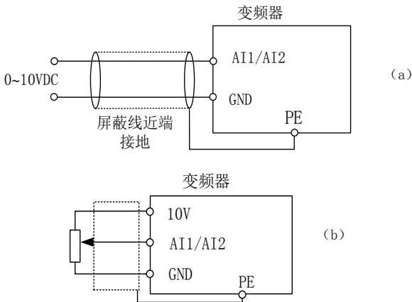
图 3-6 AI1、AI2 端子配线图
