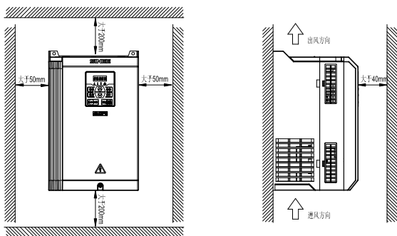
图 2-2 变频器安装方向和空间
