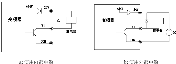
图 3-8 多功能输出端子接线方式
