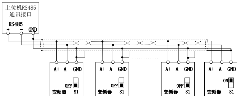
图 3-9 多台/单台变频器通讯端子配线
