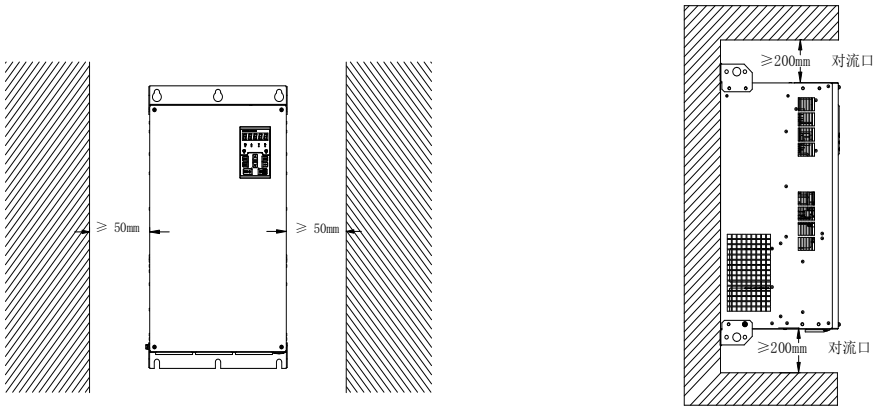
a.90~160kw 安装空间
