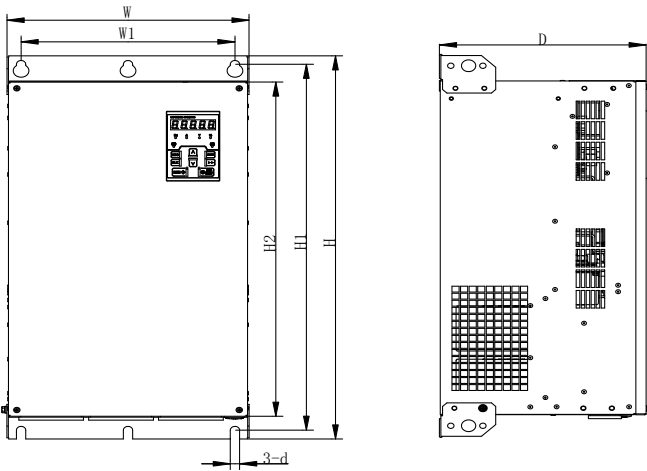
(b) 90kW~160kW 变频器外形
