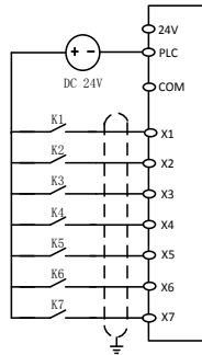
图 3-6 多功能输入端子接线图
