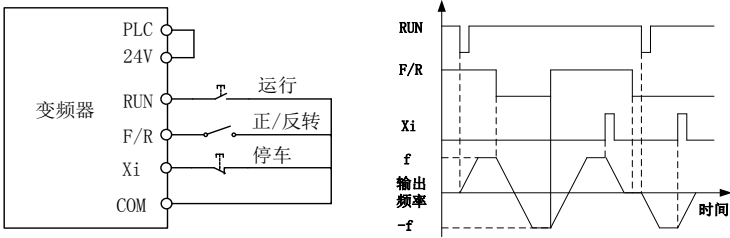
(c) F00.03=3 三线控制接线示意图 (d) F04.19=0, F00.03=3 正/反转运行逻辑 图 5-3 三线控制
