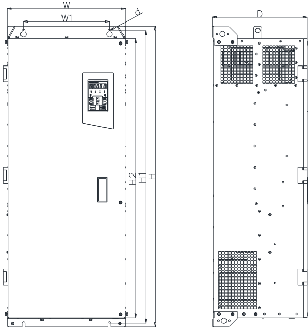
(C) 185kW~400kW 变频器外形
