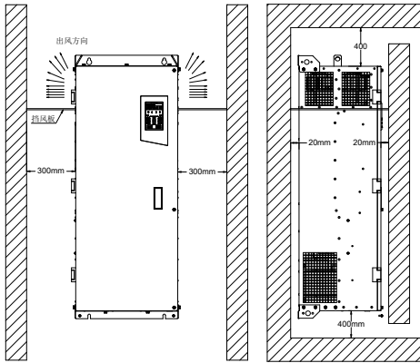
b.185~400kw 安装空间
