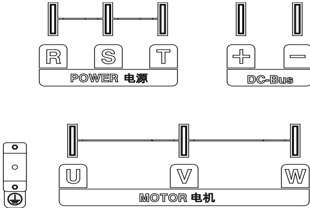
b) 132-220kW 主回路端子示意图
