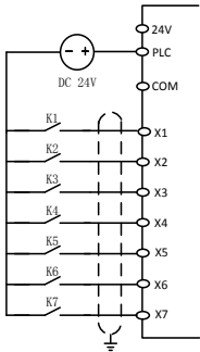
C、NPN 模式使用外部电源
