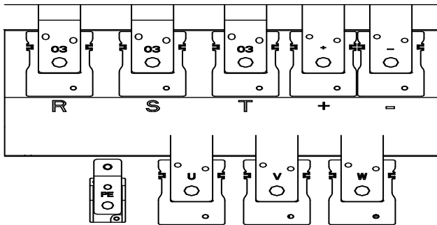
b) 132-220kW 主回路端子示意图
