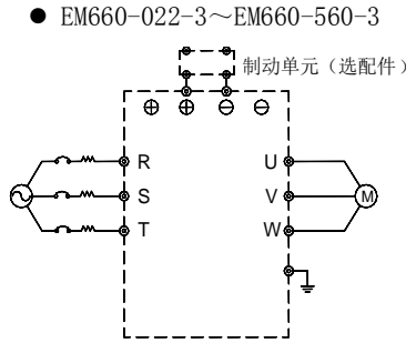
图 3-3 主回路标准接线
