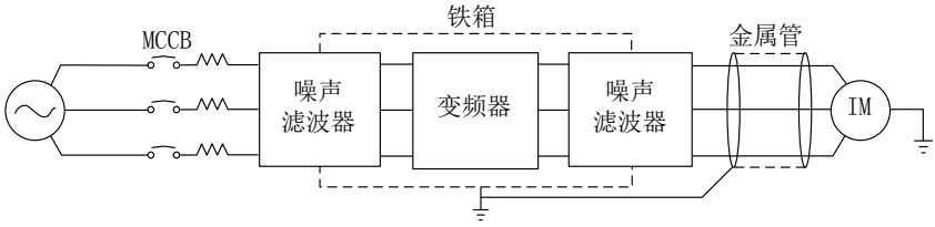
图 3-4 减少对外干扰的对策
