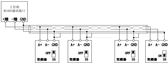
图 3-12 多台变频器通讯端子配线
