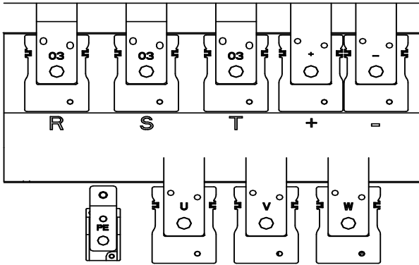
b) 132-220kW 主回路端子示意图
