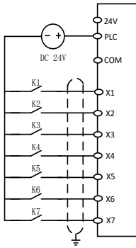
C、NPN 模式使用外部电源
