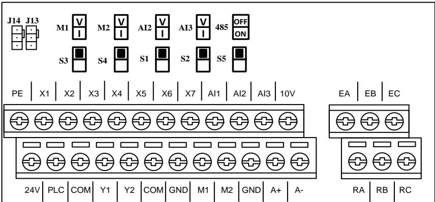
图 3-5 控制回路端子排列
