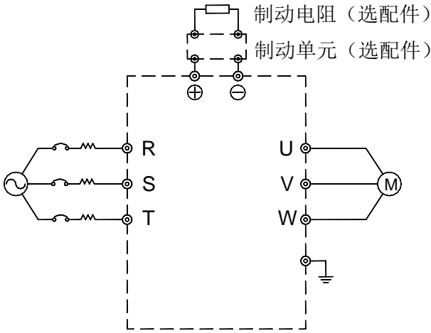
图 3-3 主回路标准接线
