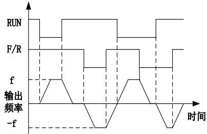
(d) F04.19=0, F00.03=1 正/反转运行逻辑
