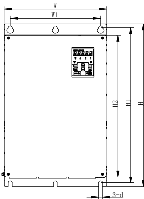
(b) 90kW~160kW 变频器外形
