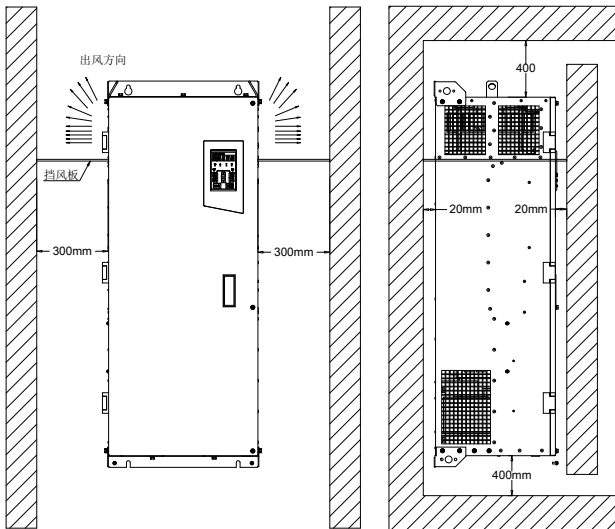
图 2-2 变频器安装方向和空间
