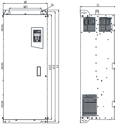
(c) 185kW~400kW 变频器外形
