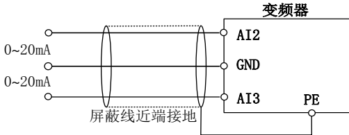
图 3-8 AI2、AI3 端子配线图
