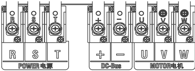
a) 90-110Kw 主回路端子示意图
