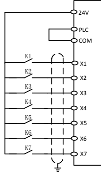
D、PNP 模式使用外部电源
