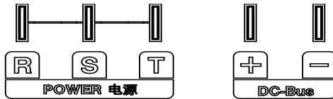
b) 132-220kW 主回路端子示意图
