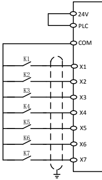
C、NPN 模式使用外部电源
