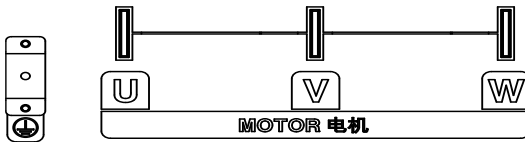
c) 250-280kW 主回路端子示意图
