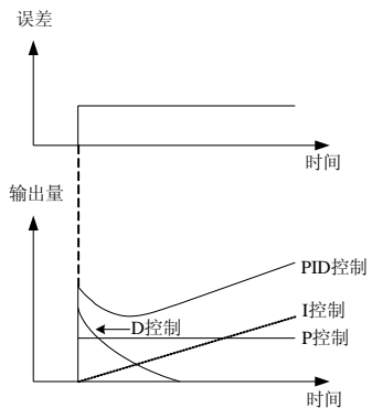
图6-25 PID控制的作用
