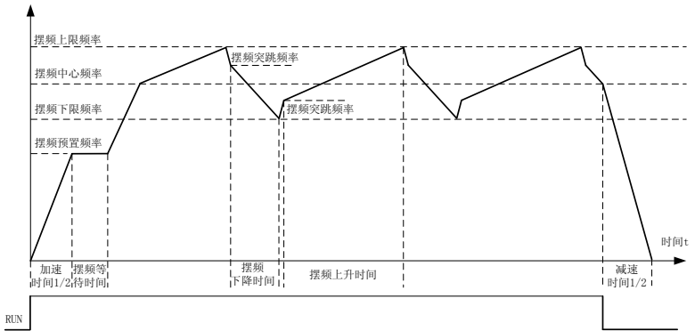
图 6-18 摆频运行逻辑图
