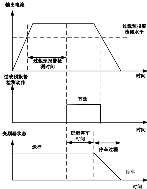
图 6-23 过载预警控制示意图
