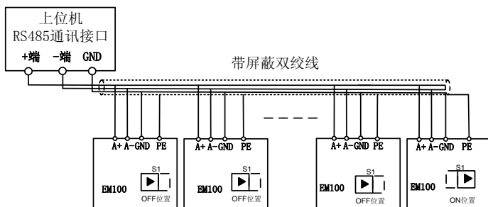
图 3-20 RS485 多点连接方式
